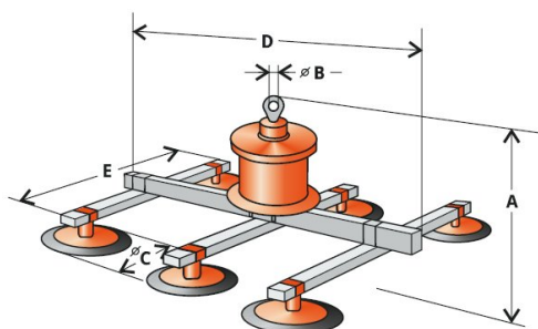
VMS 600-2
