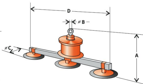
VMS 600-3
