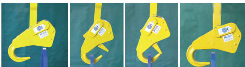
Hák zavěšený v jeřábovém háku najíždí do oka břemena.
