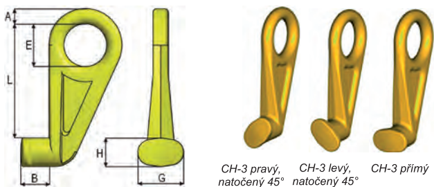
Kontejnerový hák CH-3 pravý, natočený 45°
