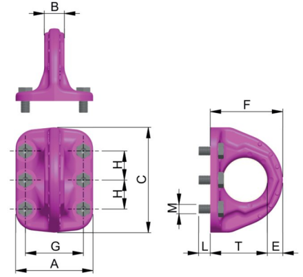
B-ABA 20 t - 31,5 t
