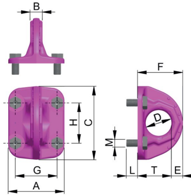
B-ABA 1,6 t - 10 t
