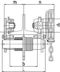
Z420-A(B) nosnost 1 t
