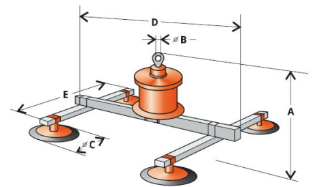
VMS 600-4 a VMS 1200-4
